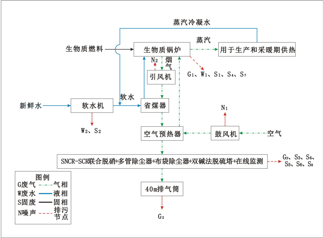
图 2-2 本项目生产工艺流程及产排污节点图
