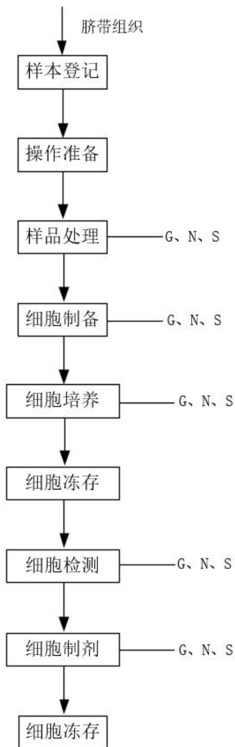
图 2-4 MSC 细胞研发工艺流程及排污节点图
