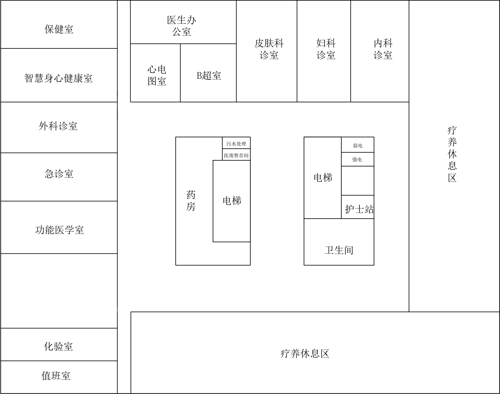
附图5 平面布置图（四层）
