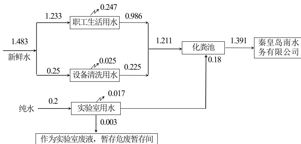
图 2-1 本项目水平衡 单位：m 3 /d
